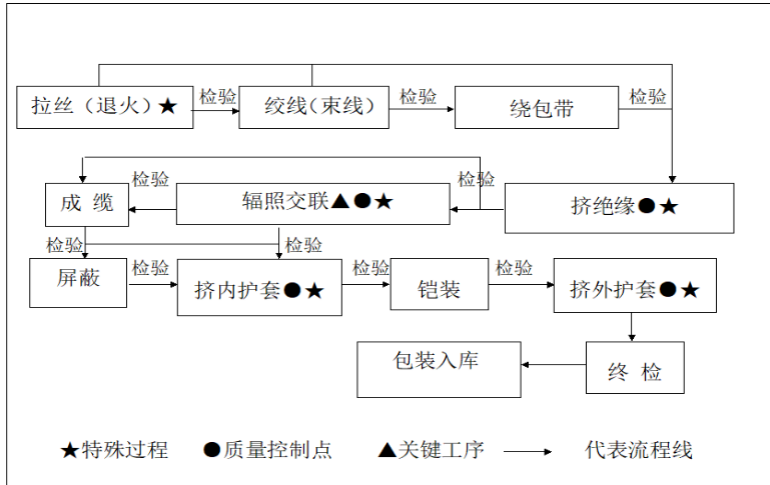
图 3-4 塑料绝缘控制电缆工艺流程图
