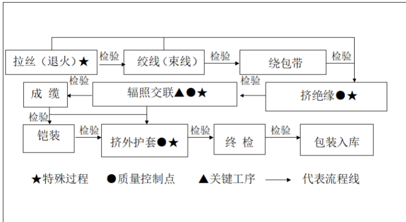
图 3-2 低压电力电缆工艺流程图
