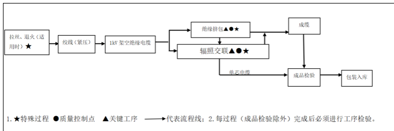
图 3-3 1kV 架空绝缘电缆工艺流程图
